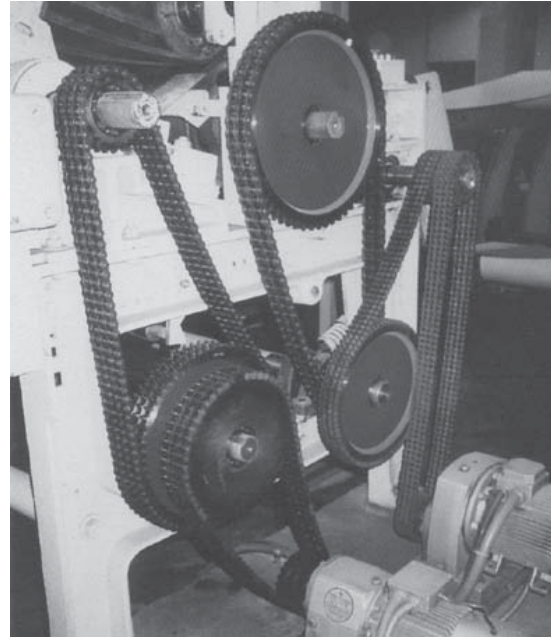
Intricado conjunto motriz con transmisiones compuestas (a contraejes) y cadenas de hilera múltiple que ejecutan variadas funciones y reducen drásticamente velocidades aún después de los moto reductores en una "convertidora de papel".
