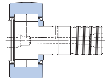
NUKR..A
