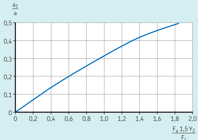
Distancia del punto donde actúa la carga radial
