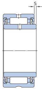
NA 49 ...2RS
