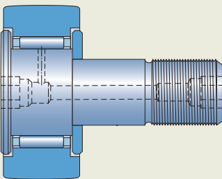
Diseño KR ..B, tamaños 22 y 26
