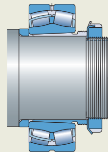
Manguito de desmontaje sobre un eje escalonado
