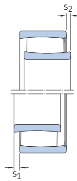
Completamente lleno
