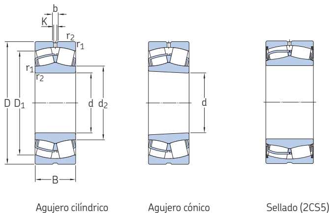
Agujero cilíndrico
